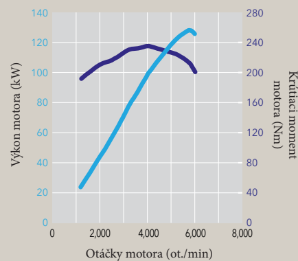
2,5-LITROVÝ MOTOR SUBARU BOXER S ROZVODOM DOHC
