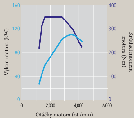
2,0-LITROVÝ PREPLŇOVANÝ VZNETOVÝ MOTOR SUBARU BOXER S ROZVODOM DOHC
